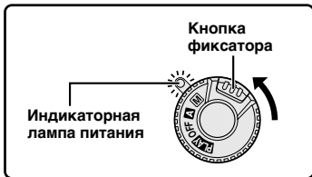
Переключатель питания
